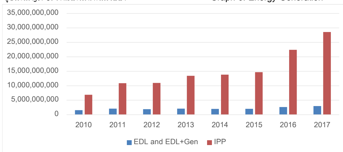
ຮູບສະແດງທີ 6: ການຜະລິດກະແສໄຟຟ້າ
